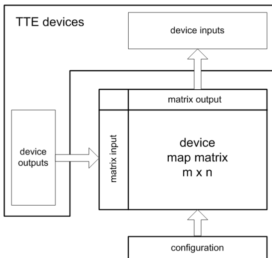
Fig. 2: Schema of TTE device „Device Map Matrix“
